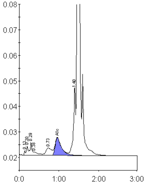
Peak table - ID: 10539835
